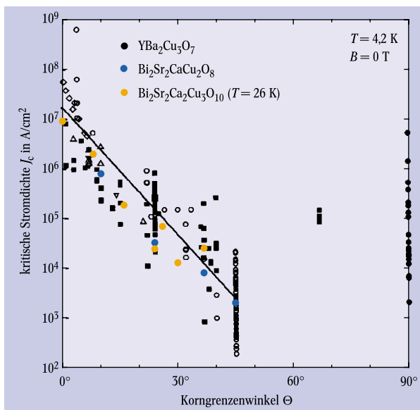
Abb. 8: Die kritische Stromdichte hängt stark von dem Verkipfungswinkel der Korngrenze von bi-kristallinen YBCO-Schichten ab. Daher muss für eine gute Stromleitung auch innerhalb der (a,b)-Ebenen eine Textur vorliegen. (Bi2212: [16], YBCO: [17], Bi2223: [18])
