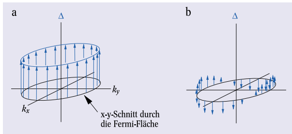
Abb. 1: Die Gap-Funktion \Delta(k_F) , der Ordnungsparameter der Supraleitung, spiegelt die Geometrie der Fermi-Fläche wider und erlaubt wichtige Rückschlüsse auf den zugrunde liegenden Supraleitungsmechanismus. |\Delta(k_F)| ist die Energielücke.
